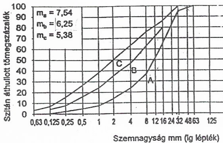
D = 32 mm-es adalékanyag szemeloszlásai
