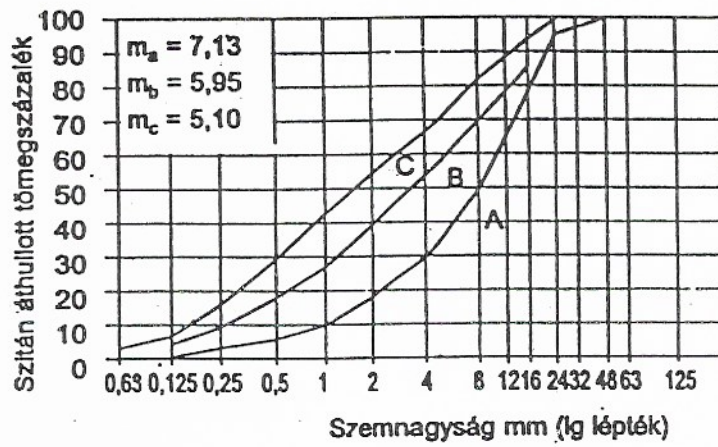
D = 24 mm-es adalékanyag szemeloszlásai
