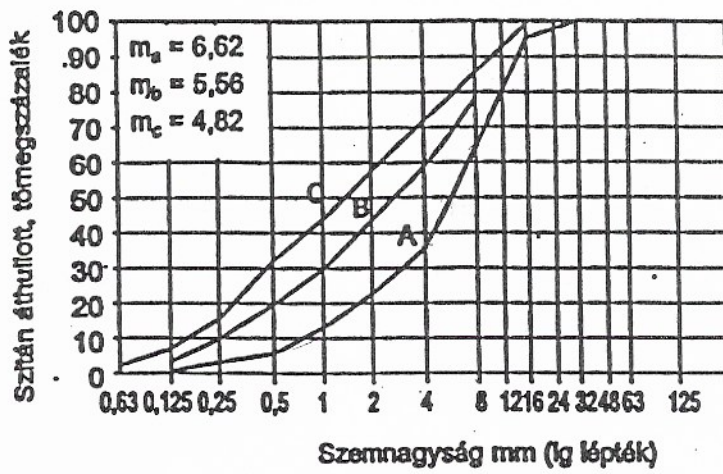
D = 16 mm-es adalékanyag szemeloszlásai
